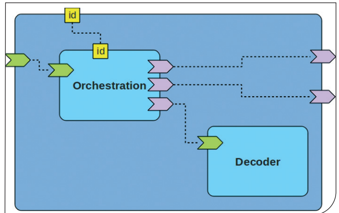
Figure 1: Implémentation du composant de décodage
